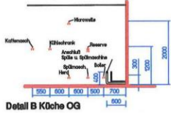
Detail B Küche OG
