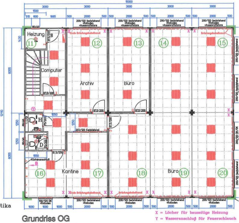
Grundriss OG
